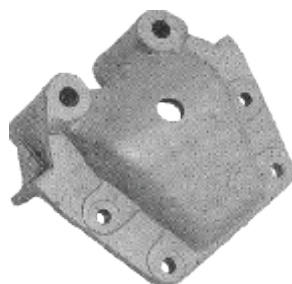
SUPORE DA MOLA TRAS. P/ DIANT. ONIBUS B-58
